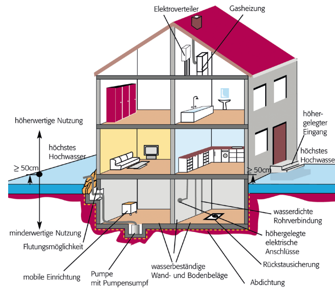
Bauliche Vorsorgemaßnahmen gegen Hochwasser (Quelle: „Hochwasserschutzfibel“, BMVBS 2002)
